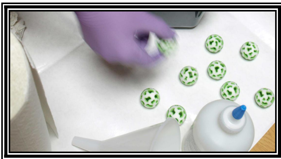
Тродимензионални модел сфере са отворима на површини и унутрашњом шупљином. Истовремено штампано више модела на 3D колор штампачу ZPrinter 250
