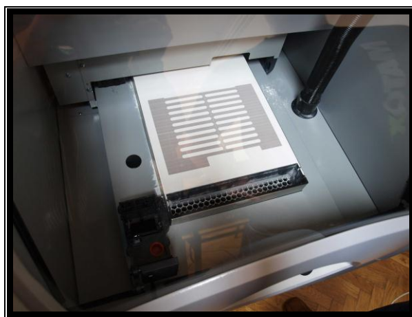
Припрема модела за штампање подешавањем параметара у програму ZPrint и ZEdit Pro и припрема штампача за штампу
